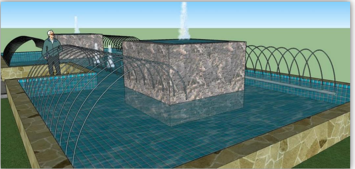
Kubbe sistemli süs havuzu 3D çizimi
