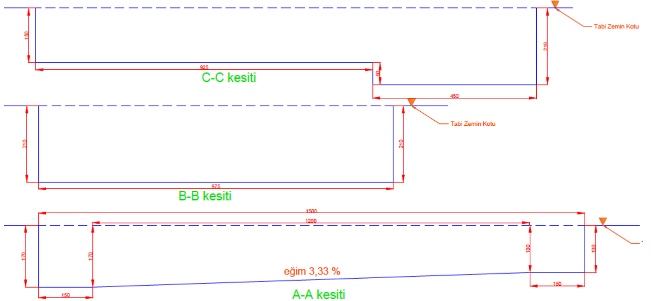
Kesit
